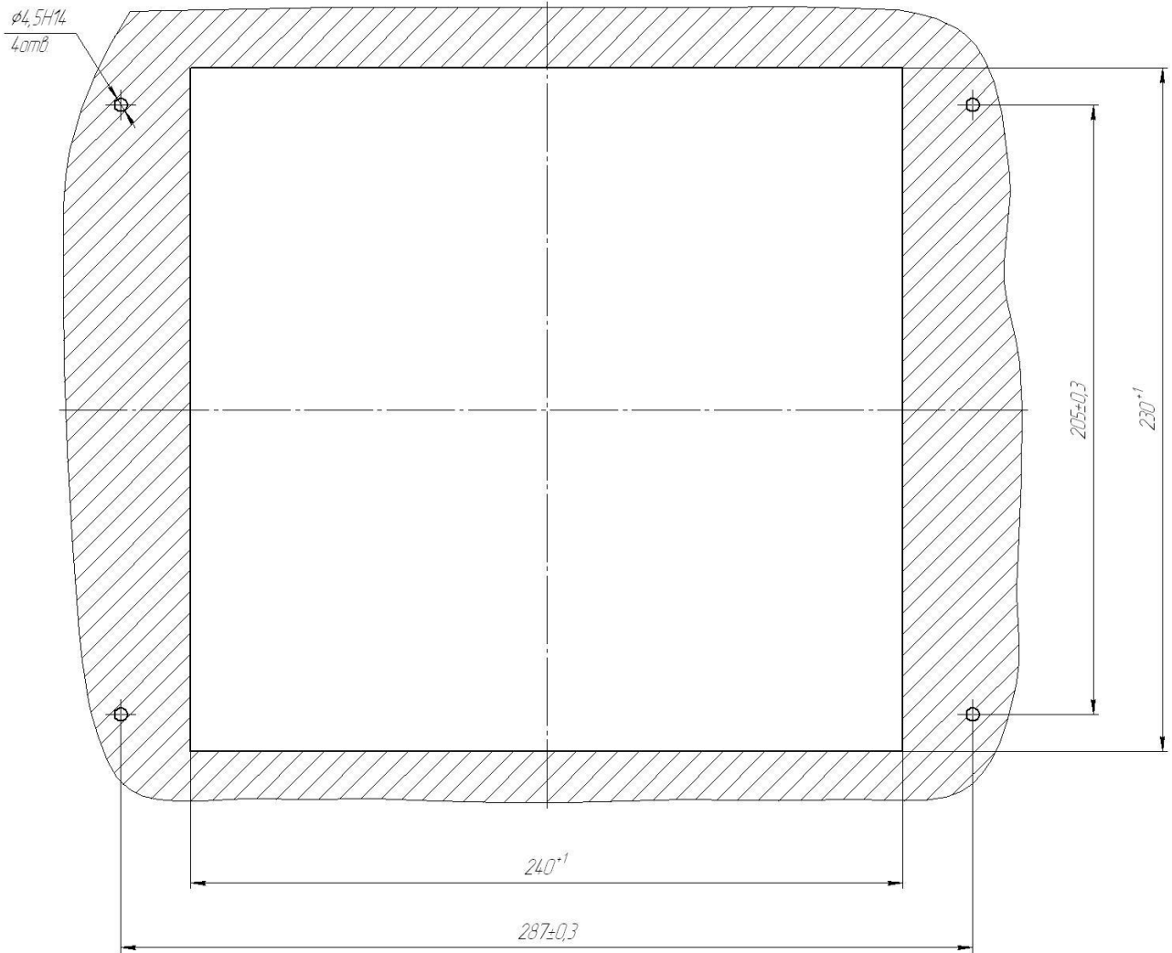
Рисунок А.5 – Габаритные размеры окна и крепежных отверстий для установки РЗЛ-05.ЦС
