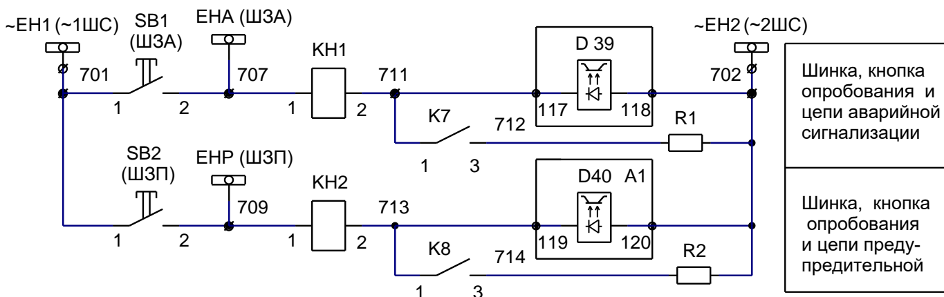
Рисунок 6б – Подключения устройства в типовую схему ЦС на переменном оперативном токе
