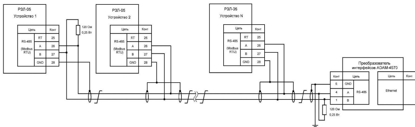
Рисунок 7 – Пример схемы организации сети с интерфейсом RS-485
